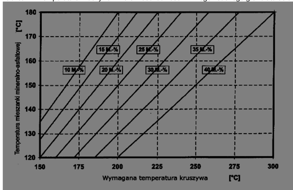
Tablica 12. Temperatura kruszywa w zależności od ilości zimnego i suchego granulatu asfaltowego
